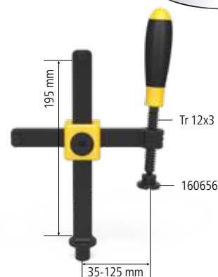
2-160610 Pince de bridage Professional - brunie / nitrurée 58,00 € •
